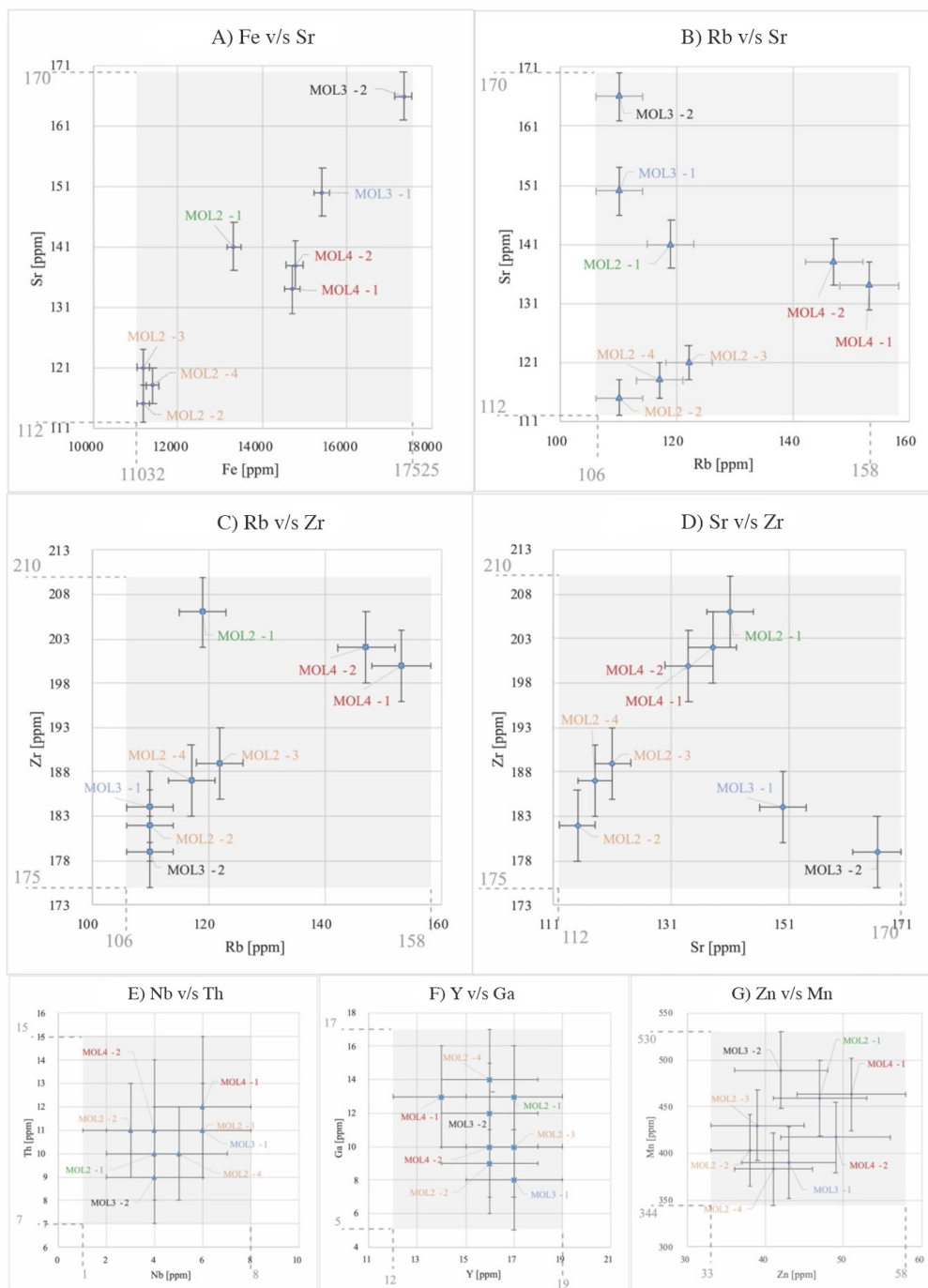
Fig. 4. Análisis FRX. Resultados de concentraciones de elementos en PPM, obtenidos de análisis FRX para las muestras de obsidiana de los sitios Moluco 2, Moluco 3 y Moluco 4. A) Fe vs Sr; B) Rb vs Sr; C) Rb vs Zr; D) Sr vs Zr, E) Nb vs Th; F) Y vs Ga y G) Zn vs Mn. Cuadros con fondo gris claro indica área de variabilidad. Gráficos A, B, C y D corresponden a elementos usados para discriminar fuentes volcánicas (Fe, Sr, Rb y Zr). Líneas muestran la desviación estándar para cada muestra. La variabilidad de los elementos de todas las muestras permite caracterizar las fuentes naturales de los Nevados de Solipulli para futuras comparaciones con métodos equivalentes.
