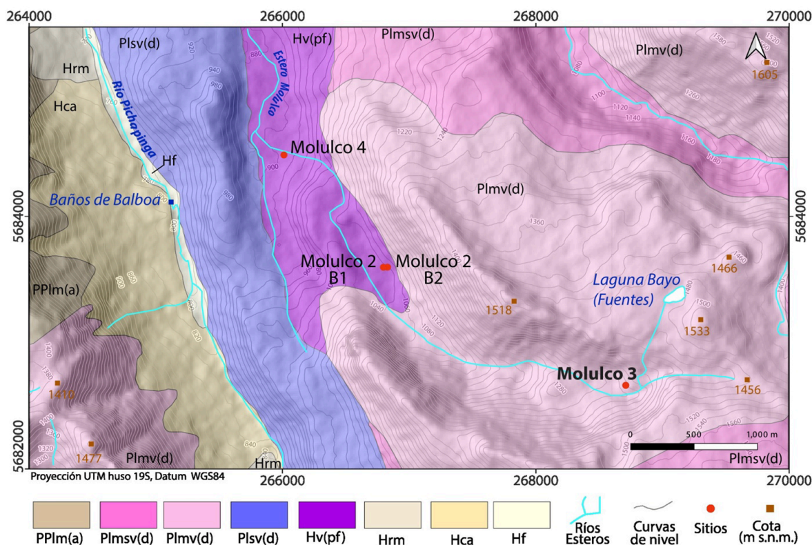
Fig. 3. Mapa geológico del área de estudio, modificado de Lemus y Honores (2019). Se observa que algunos sitios se distribuyen a lo largo del estero Molulco en las unidades geológicas Hv(pf) y Plmv(d). Laguna Fuentes corresponde a laguna Bayo según carta Melipeuco del Instituto Geográfico Militar, escala 1:50.000.
