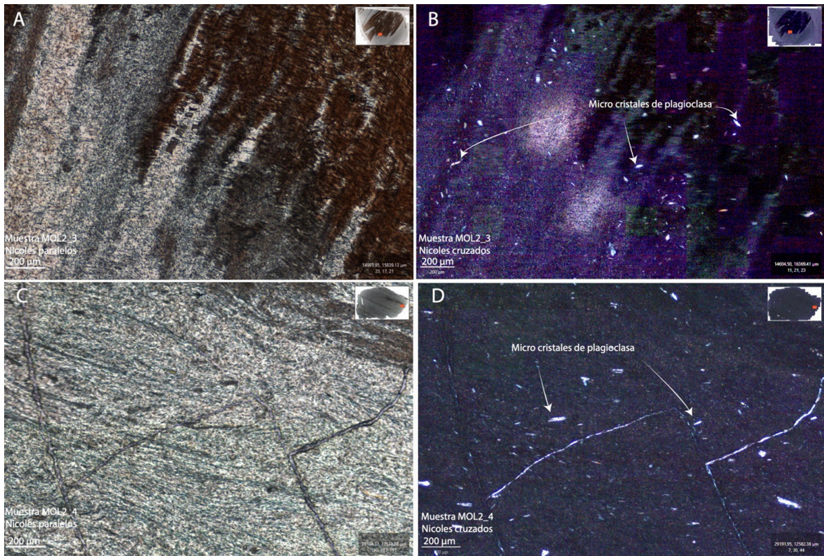
Fig. 6. Fotos de cortes transparentes para las muestras del sitio Molulco 2, Mol2-3; A) a nicoles paralelos; B) a nicoles cruzado en el mismo lugar; y Mol2-4; C) a nicoles paralelos; D) a nicoles cruzados. Notar la presencia de micro cristales de plagioclasa. Muestra Mol2-4 muestra tamaños de microcristales ligeramente más grande que para la muestra Mol2-3.
