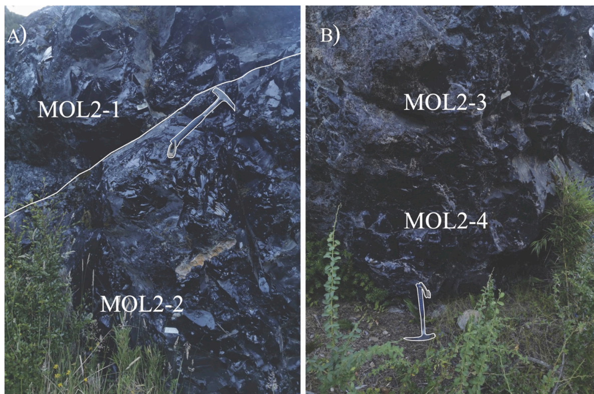
Fig. 5. Fotos de los bloques del sitio Molulco 2. A) Bloque 1 y superficie de contacto que evidencia 2 flujos de lava distintos, consistente con diferencias en análisis de FRX; B) Bloque 2, de donde se obtuvieron las muestras MOL2-3 y MOL2-4. El martillo es aproximadamente de 30 cm de largo.
